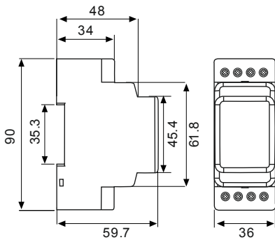
Size (Type PK 28)
